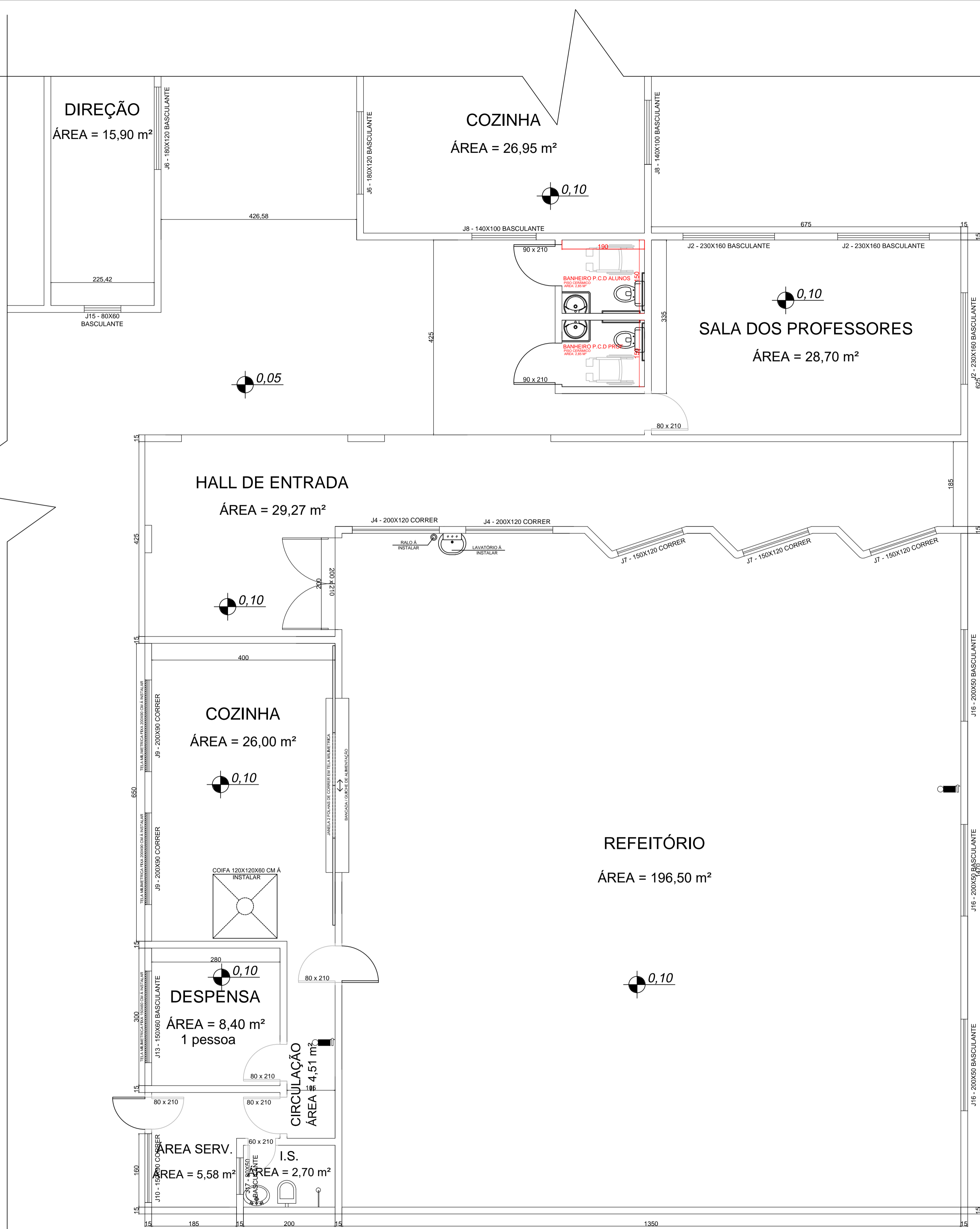
PLANTA BAIXA DESEJADA ESCALA:
